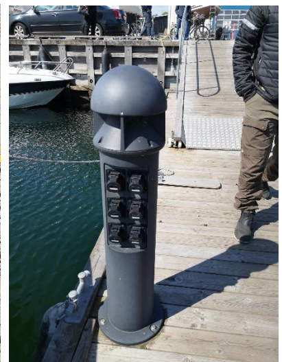
Der er indkøbt nye forsyningsstandere med el. Standerne forsynes med betalingsmoduler til el og vand.
